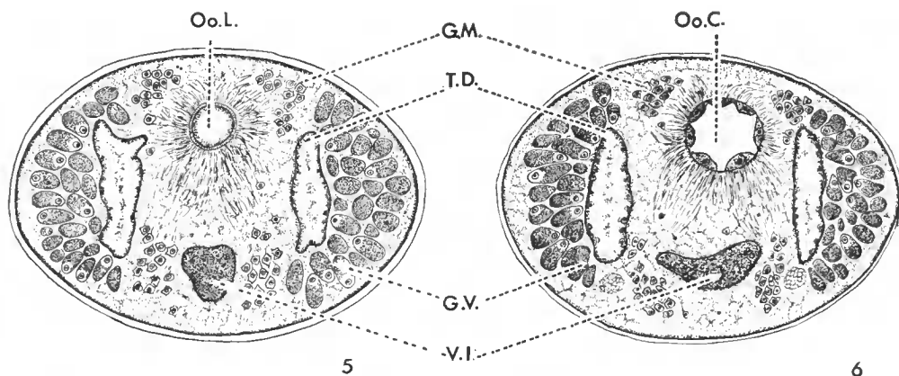
FIG. 5. — Schéma d'une coupe histologique d'un Epicotyle n. g.
